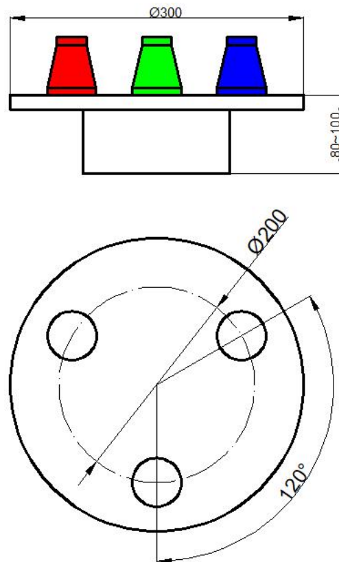
图 2 原料区示意图
